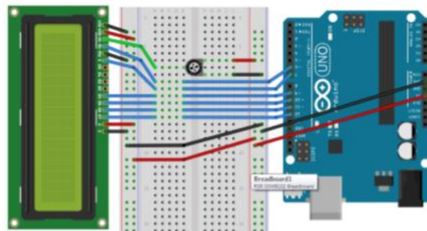
Gambar 7 Rangkaian Dasar LCD
