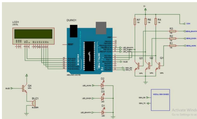
Gambar 8 Skema ADEBA
